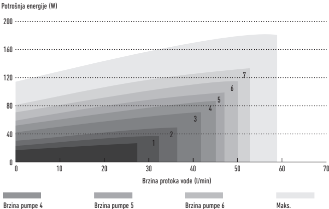
Učinkovitost hidrauličke pumpe za toplinske pumpe tipa F: Pumpa F klase A (5 kW i 16 kW).
