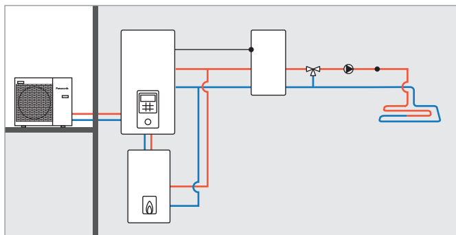
Aquarea generacije H: Bivalentno s međupremnikom i ventilom za miješanje.
