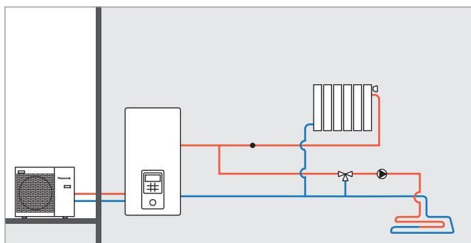
Aquarea generacije H: 2 zone s vanjskim kompletom bez međupremnika.
