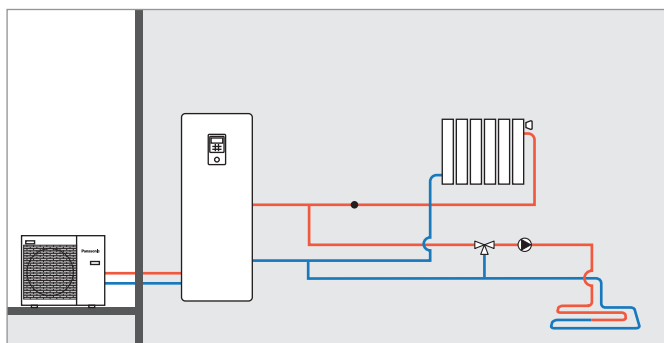
Aquarea All in One generacije G: 2 zone s vanjskim kompletom, bez međupremnika.
